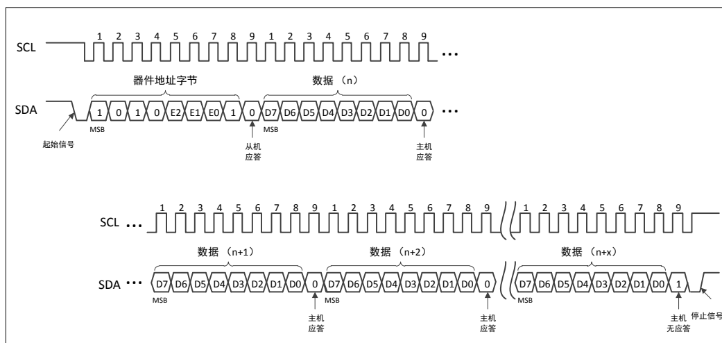
图 5-11 连续读取
