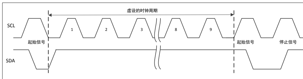
图 3-2 2 线软复位示意图
