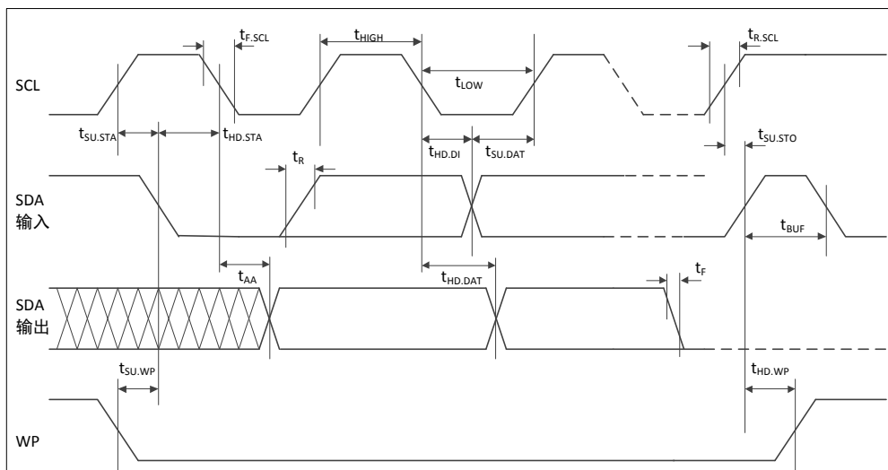
图 6-1 总线时序
