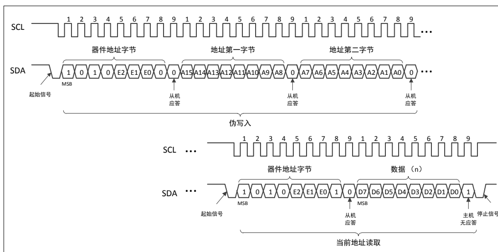
图 5-10 随机读取
