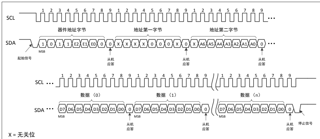
图 5-7 写入标识页
