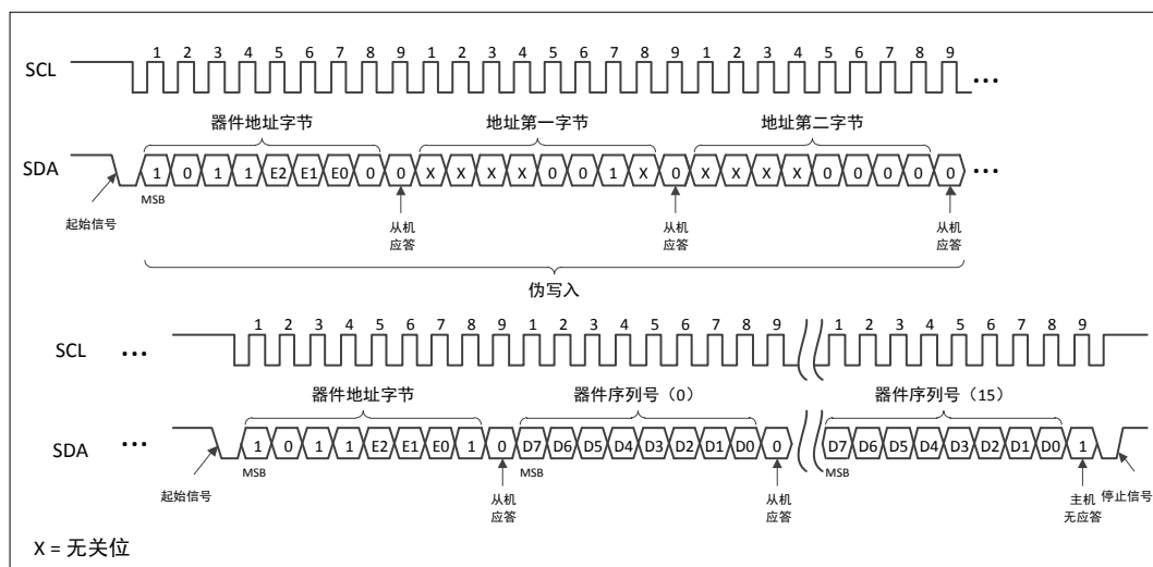
图 5-14 读取器件序列号
