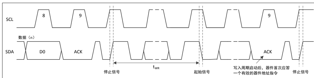
图 5-5 写入周期定时
