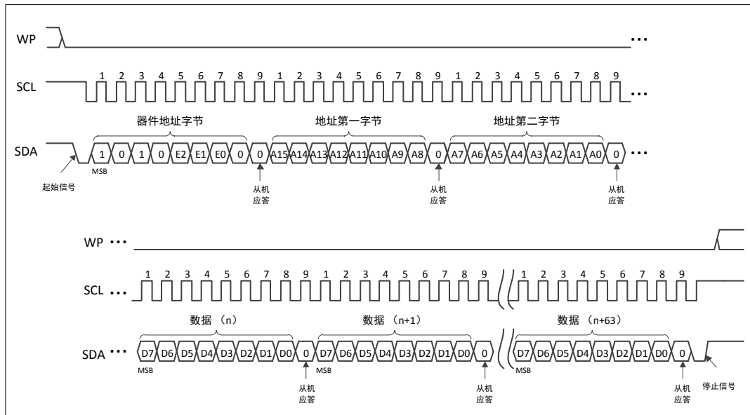
图 5-3 页写入，写保护引脚置为低
