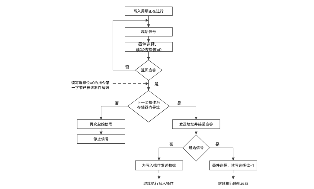
图 5-6 应答查询流程图
