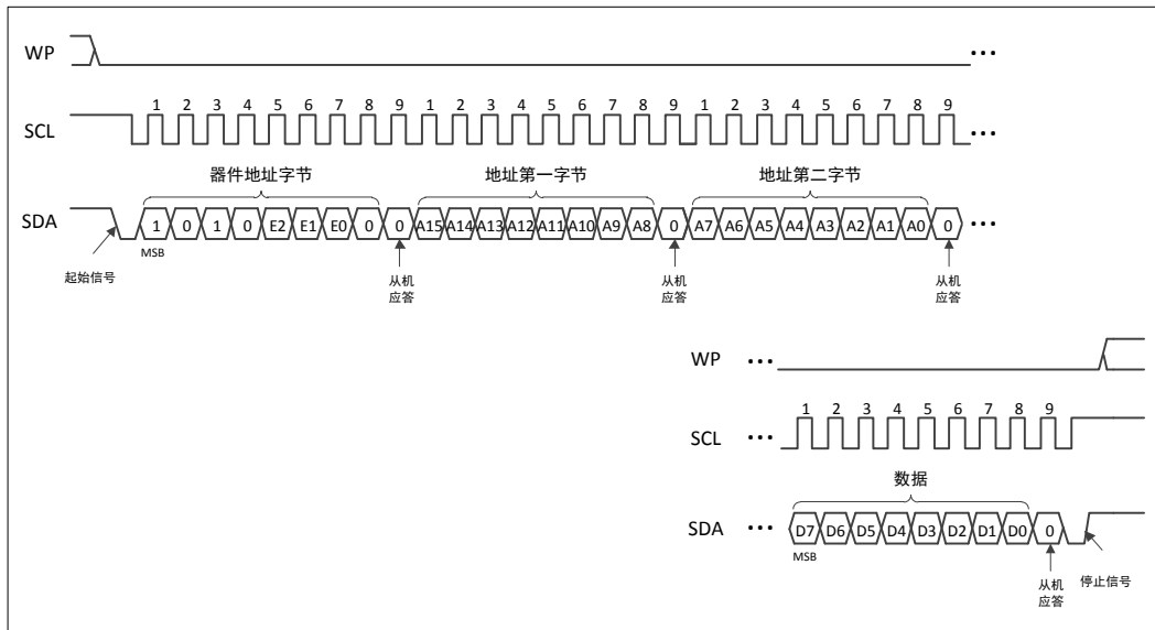
图 5-1 字节写入，写保护引脚置为低
