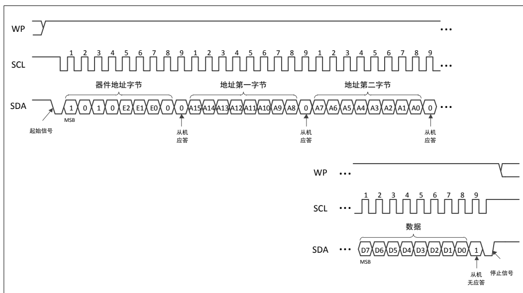
图 5-2 字节写入，写保护引脚置为高
