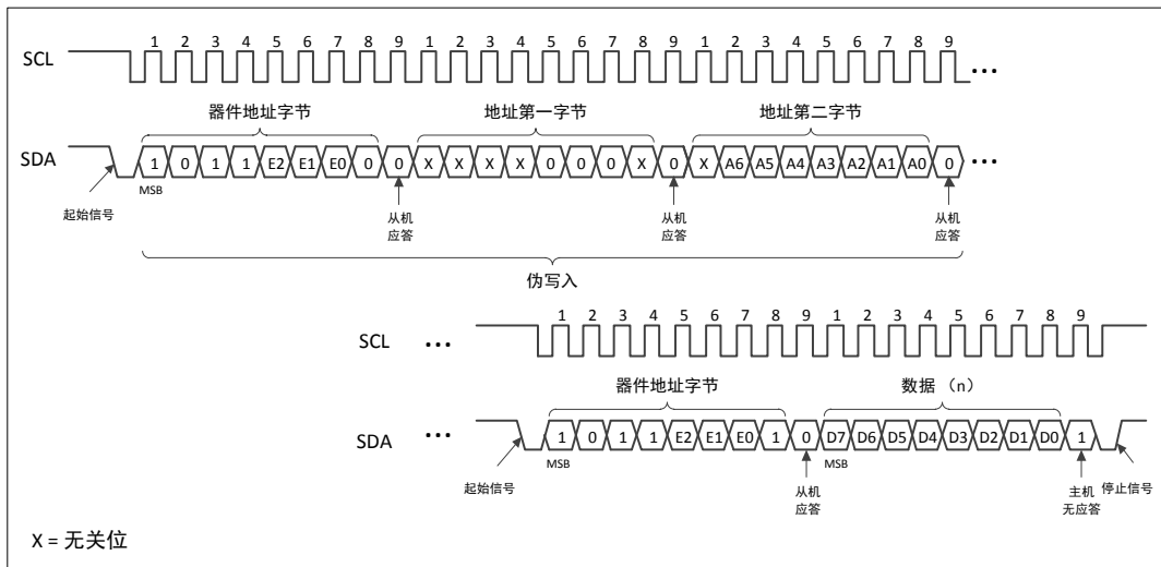
图 5-12 读取标识页
