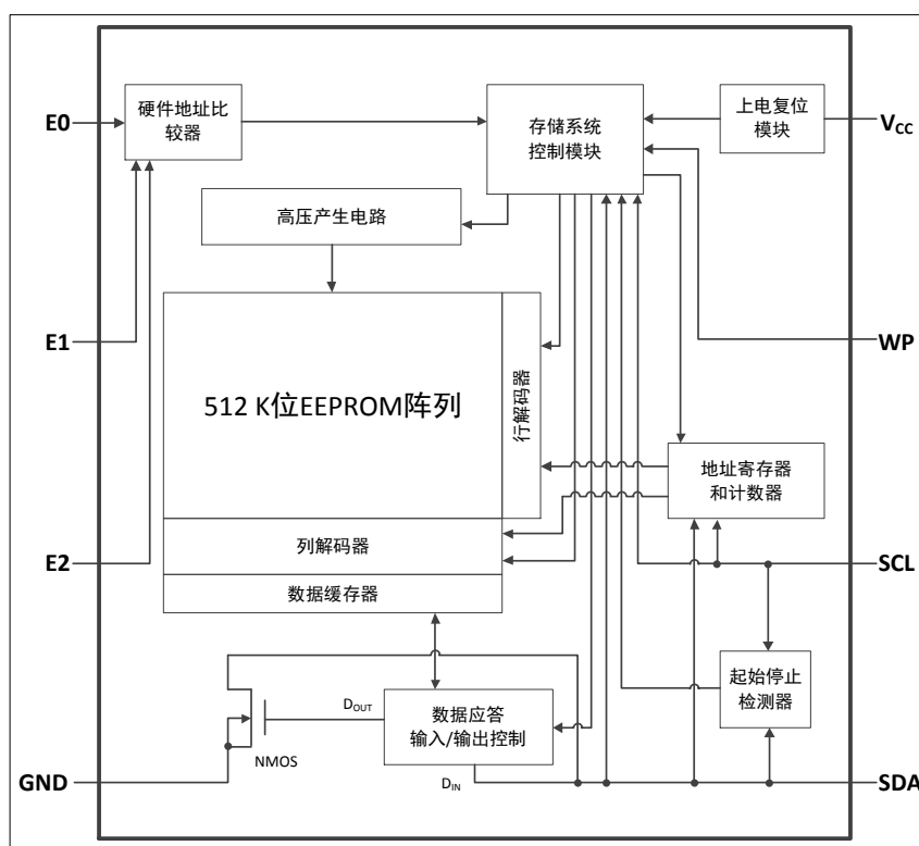
图 2-1 功能框图
