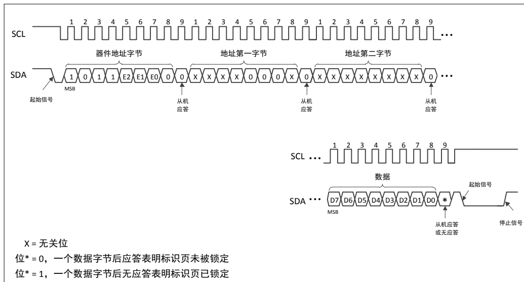
图 5-13 读取锁定状态
