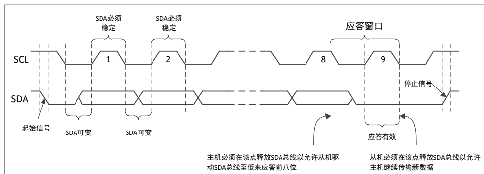
图 3-1 起始信号、停止信号和应答
