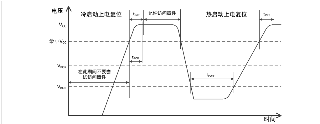
图 3-3 上电和下电时序图
