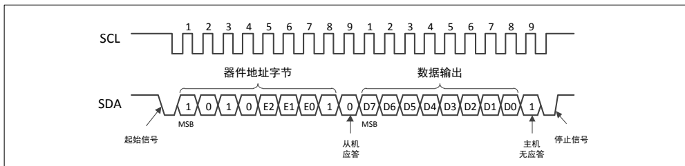
图 5-9 当前地址读取
