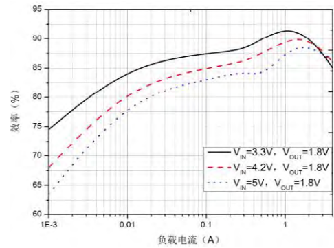
图 3 V_{OUT}=1.8V 效率
