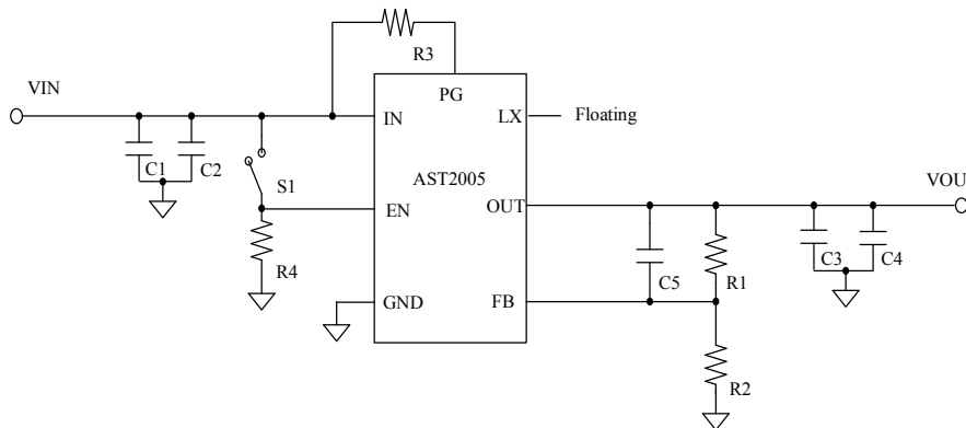
图 5 AST2005 典型应用图
