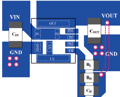
图 6 AST2005 PCB 布局示意图
