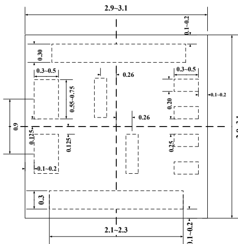
图 7 底视图
