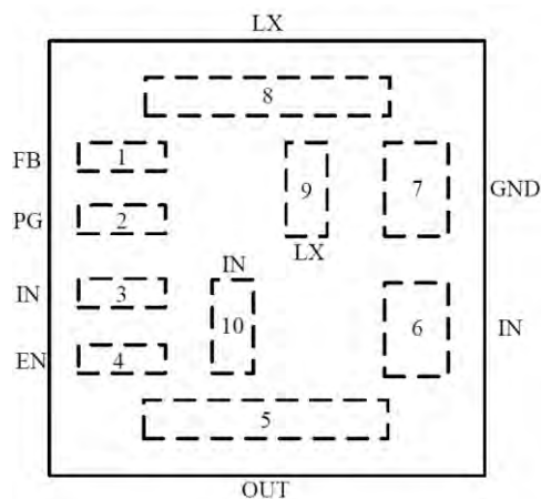
图 1 AST2005 引脚分布图（顶视图）
